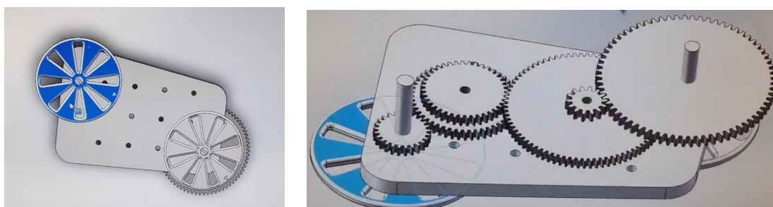
图 1-1 固定传动比齿轮系示意图
